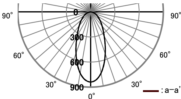
配光曲線 (cd/1000[lm])
