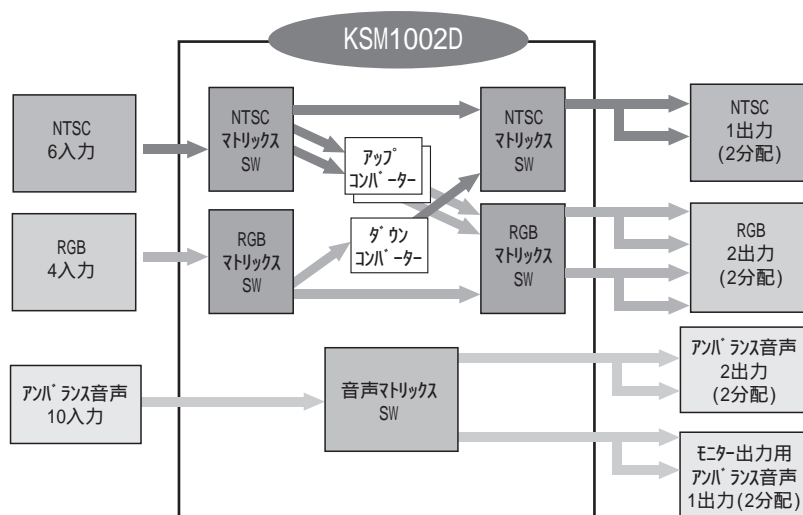
KSM1002D ブロック図
