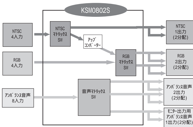
KSM0802S ブロック図
