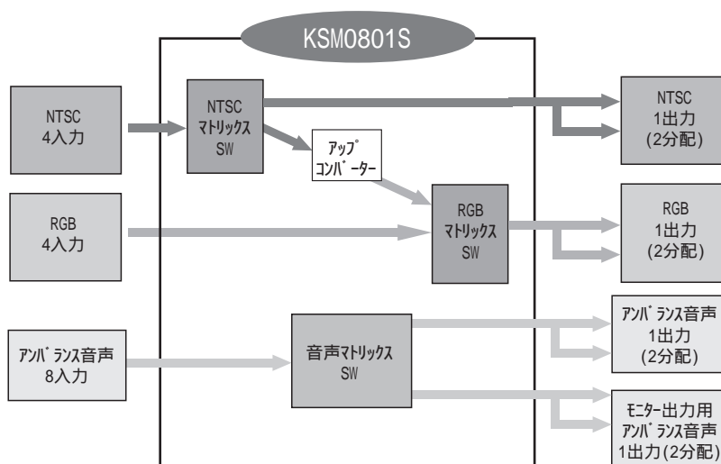
KSM0801S ブロック図
